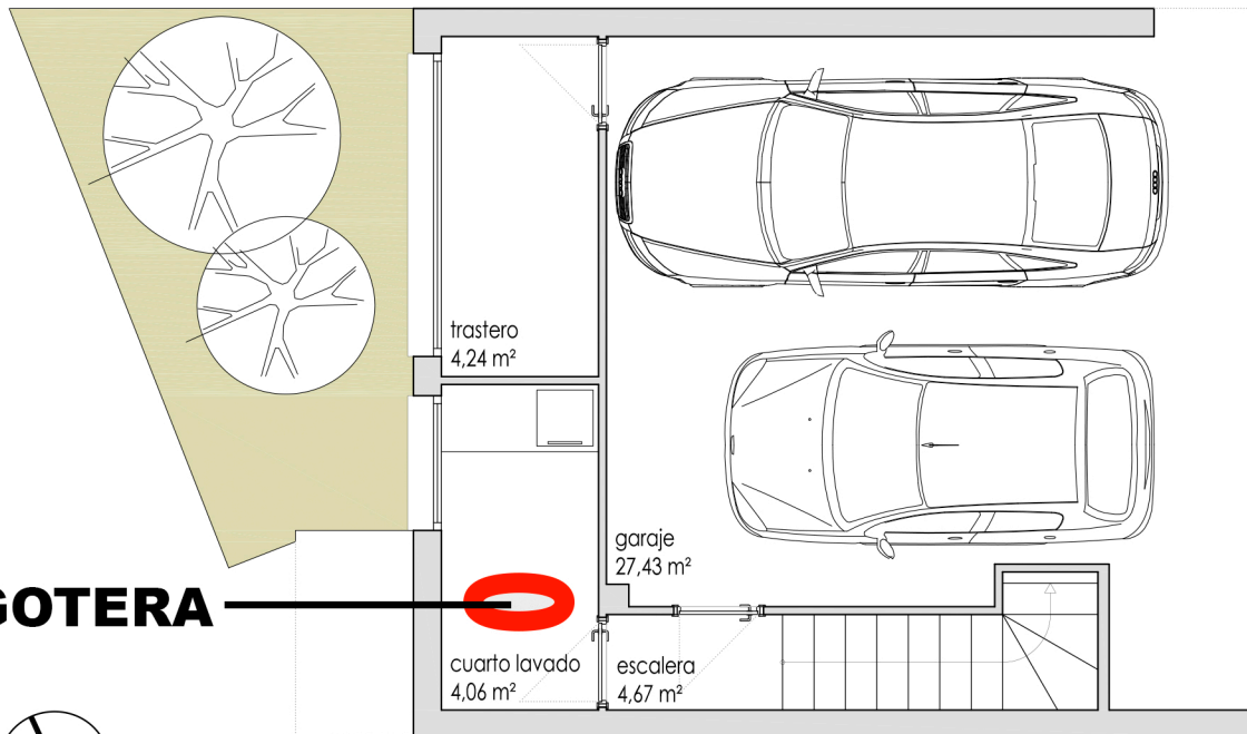
PLANTA SÓTANO
